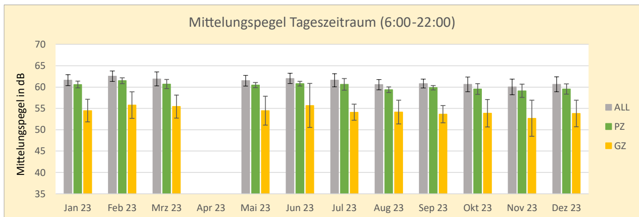
Abbildung 5. Mittelungspegel des Tagzeitraums am Referenzquerschnitt des Fahrbahnlabors im Jahr 2023.
