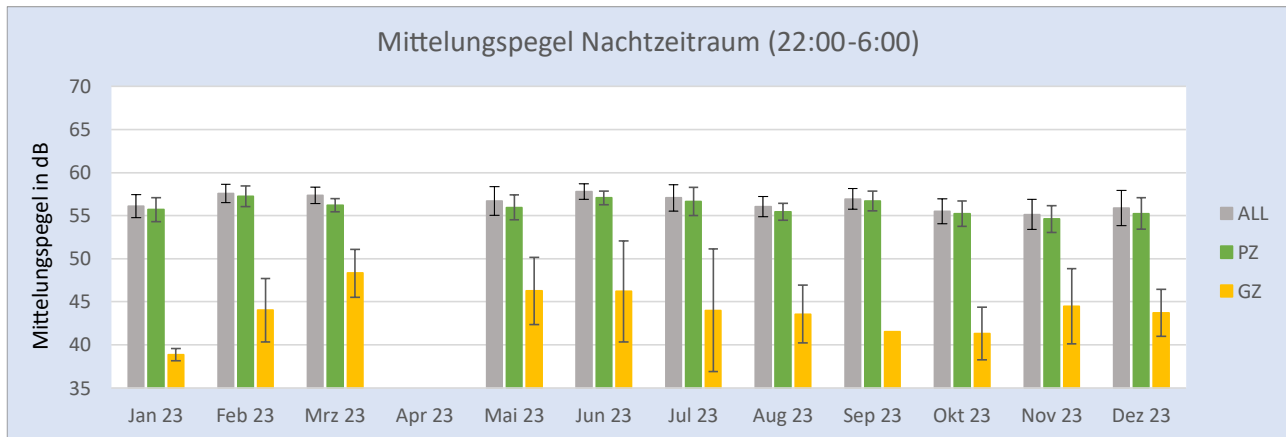
Abbildung 6. Mittelungspegel des Nachtzeitraums am Referenzquerschnitt des Fahrbahnlabors im Jahr 2023.
