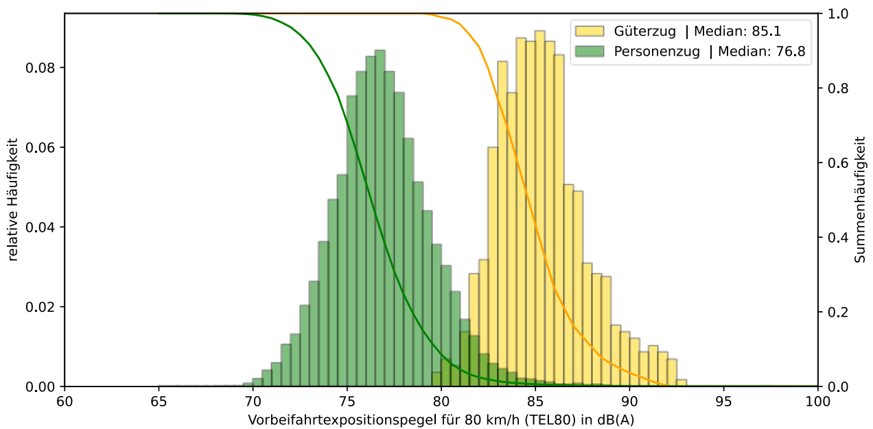
Abbildung 9. Relative Häufigkeitsverteilung und Summenhäufigkeit aller im Jahre 2023 gemessenen Vorbeifahrtexpositionspegel ( d = 7,5 m) für die Bezugsgeschwindigkeit 80 km/h, getrennt nach Güter- und Personenzügen.
