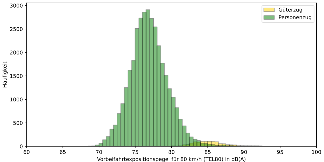
Abbildung 8. Häufigkeitsverteilung aller im Jahre 2023 gemessenen Vorbeifahrtexpositionspegel für die Bezugsgeschwindigkeit 80 km/h, getrennt nach Güter- und Personenzügen.
