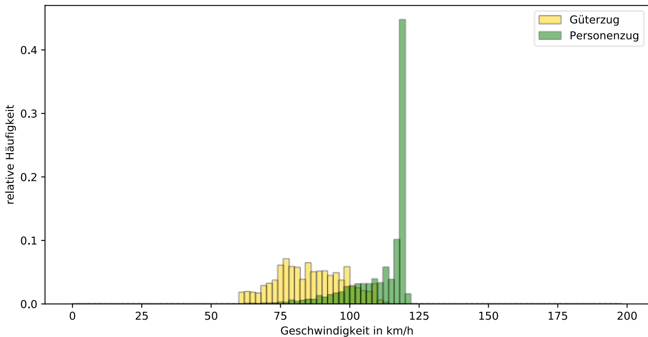
Abbildung 10. Häufigkeitsverteilung der Fahrgeschwindigkeiten der vorbeifahrenden Züge.
